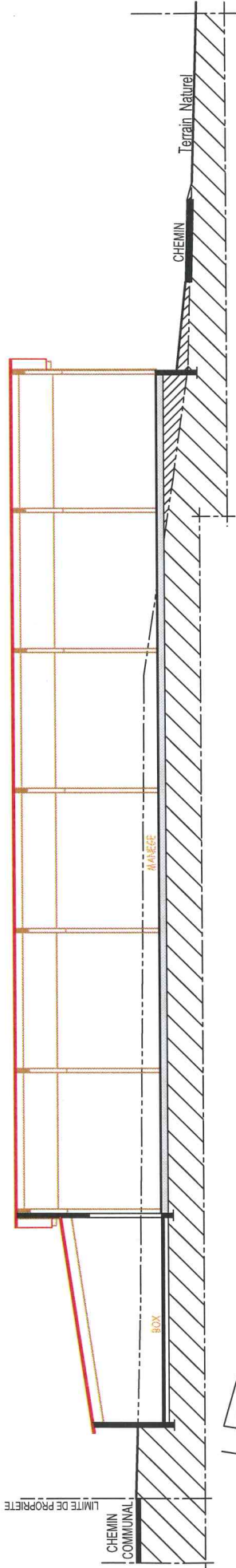
PROFIL TERRAIN Ech : 1/200°
